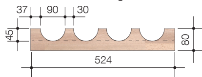
Ansicht Flaschenablage
