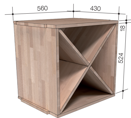
Ansicht unterer Kasten
