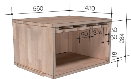
Ansicht unterer Kasten
