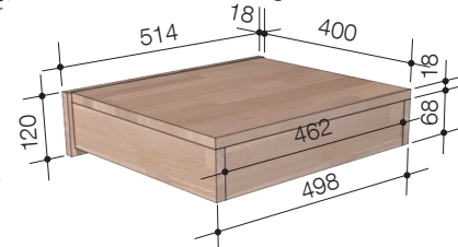
Ansicht Flaschenablage
