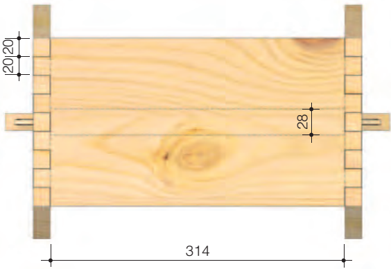
Seitenansicht
