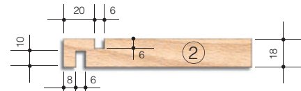
Schnitt B-B
