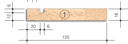
Schnitt D-D
